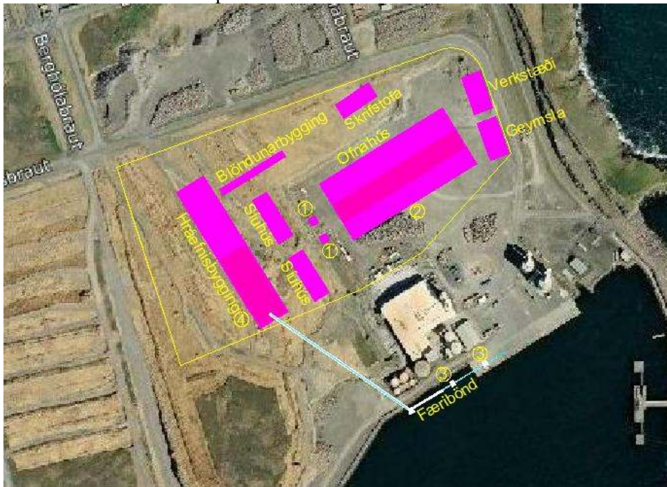
Mynd 6.10: Uppsprettur hávaða á rekstrartíma
