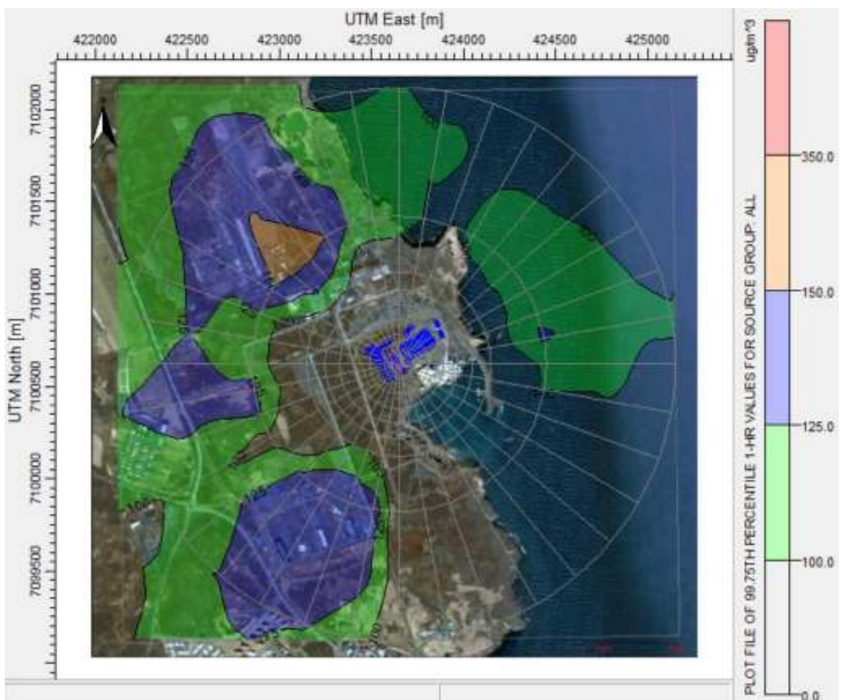
Mynd 6.3: Styrkur SO_2 á klukkustund í einingunni \mu g/m^3 (99,75 % líkan)
