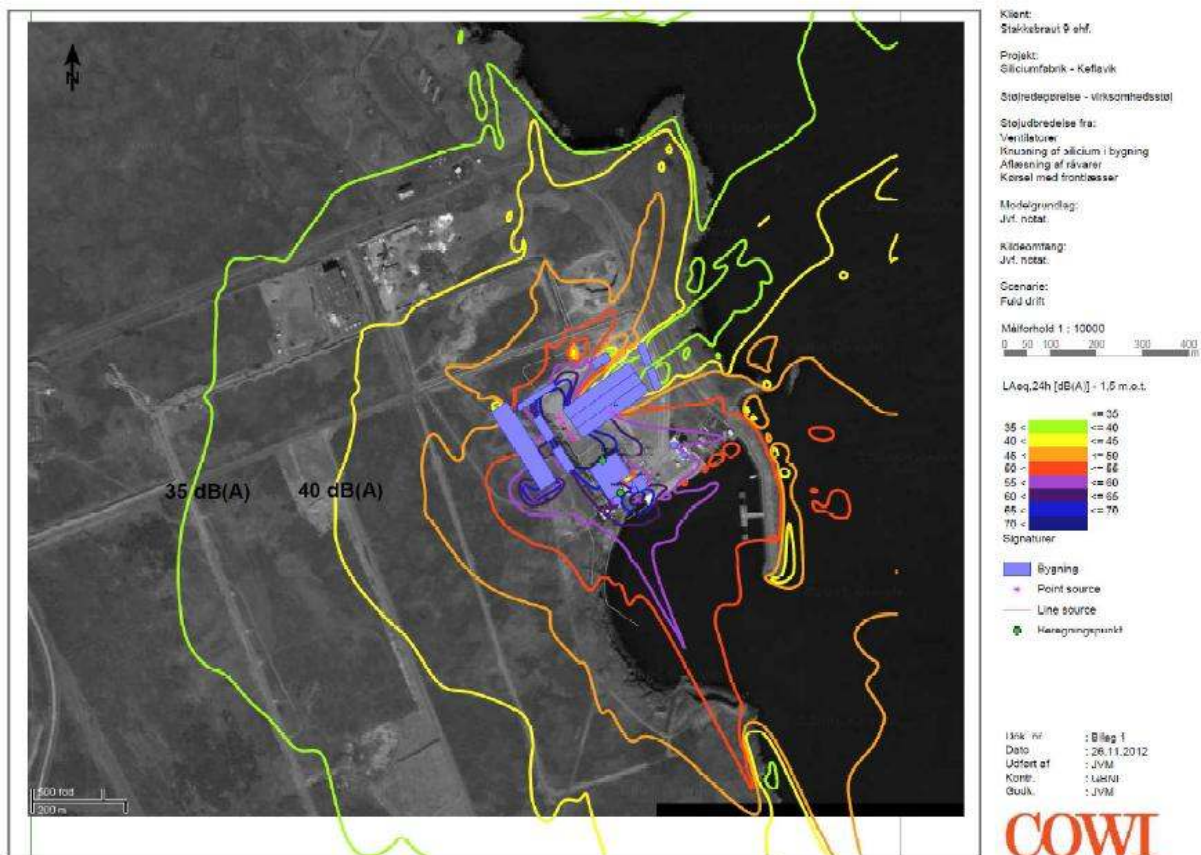
Mynd 6.11: Hljóðstig kísilverksmiðjunnar á rekstartíma
