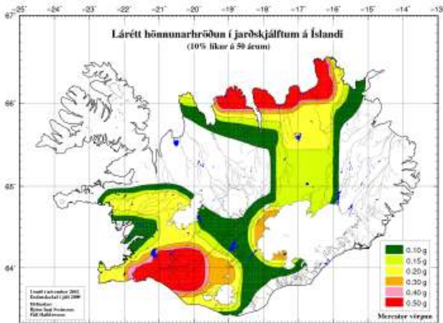
Mynd 4.2 Hröðunarkort yfir Ísland, frá árinu 2009, sem fylgir EUROCODE 8 /13/
